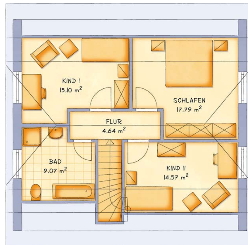
Dachgeschoss
